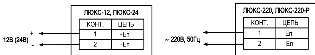
Рис.1. Схемы подключения.
