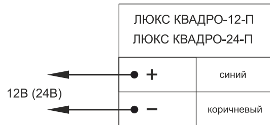
Рис.1. Схема подключения.
