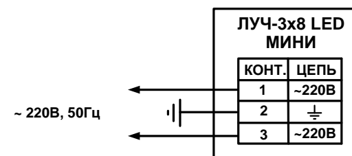
Рис. 1. Схема подключения
