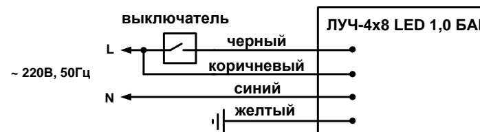
Рис.2. Схема подключения светильников непостоянного действия
