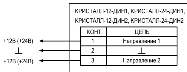
Рис.1. Схема подключения.
